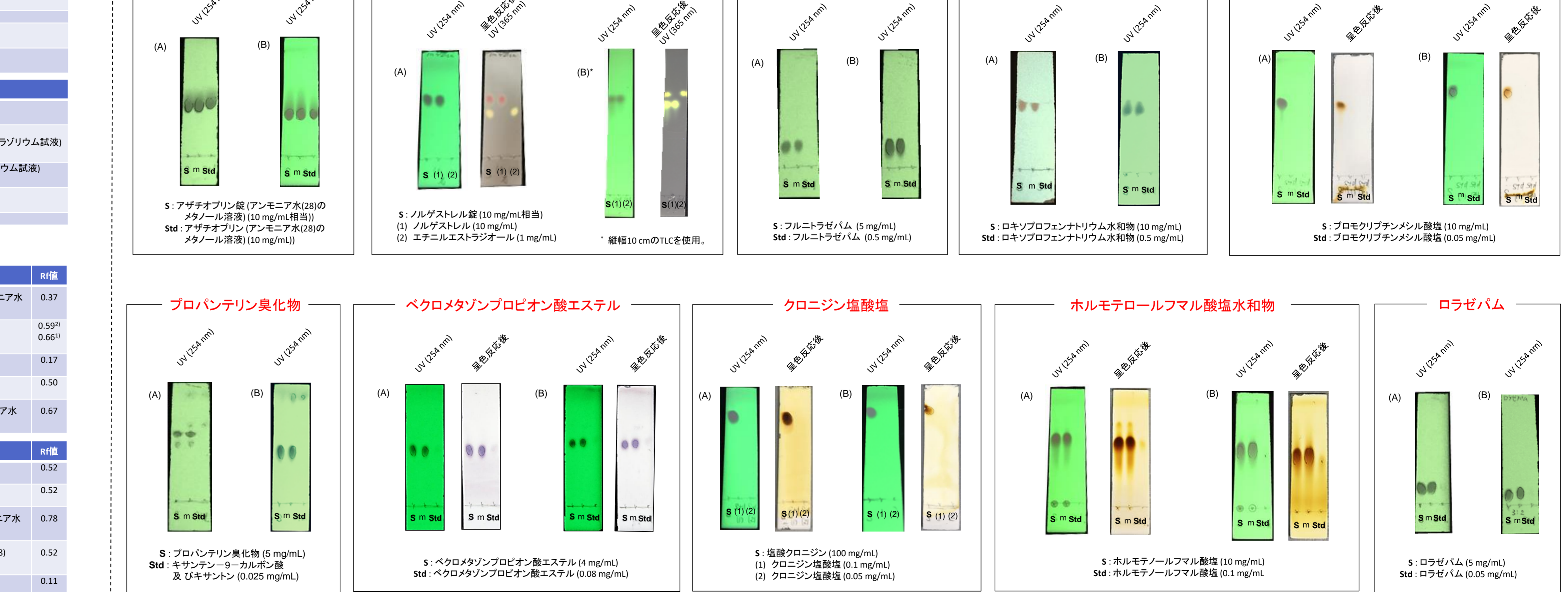
図4. TLCを用いた確認試験 (A) 現行の展開溶媒、(B) 本研究で検討した展開溶媒 (S: 試料溶液、Std: 標準溶液、m: S + Std)
