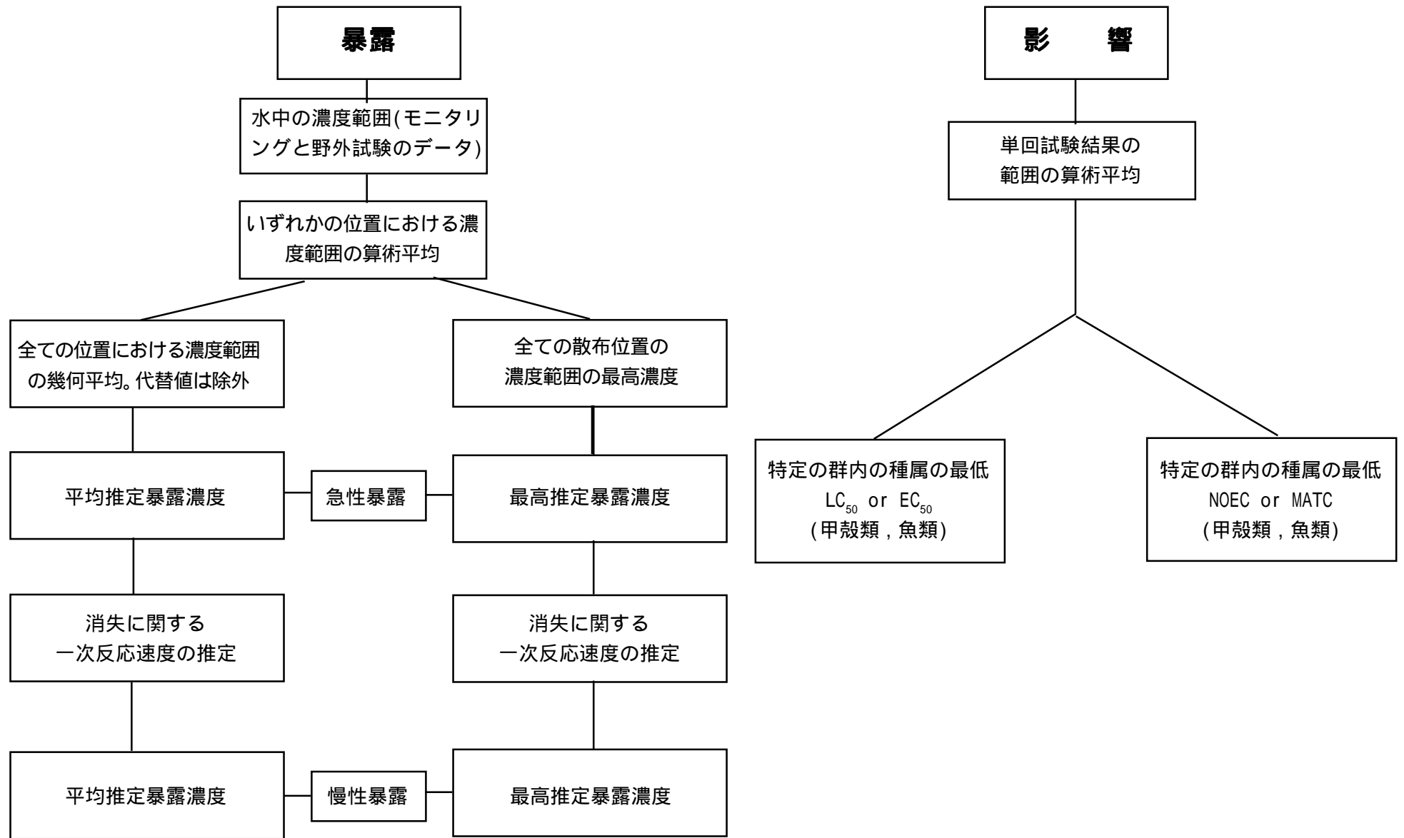
Fig. 1 暴露と影響に関する環境中濃度の推定に用いた方法
