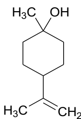
β-Terpineol
