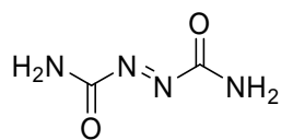
azodicarbonamide (ADC)
