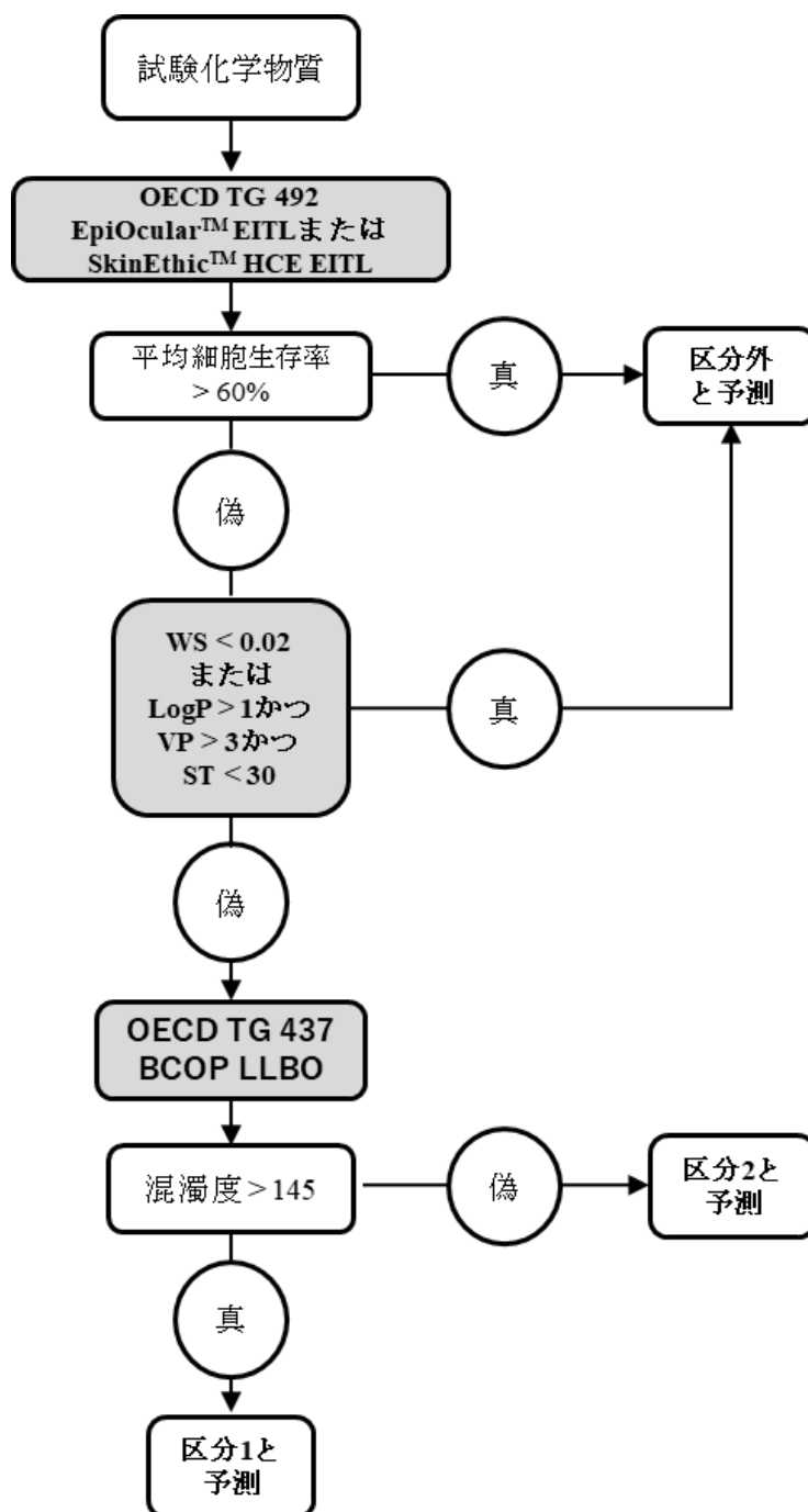
図 2.2. DAL-1 選択肢 2 の模式図。第 1 ステップ—区分外 の特定に用いる RhCE EITL 試験法。第 2 ステップ—区分外を特定する物理化学的特性の除外ルール（WS：水溶性（単位：mg/mL）か、LogP：オクタノール／水分配係数、VP：蒸気圧（単位：mm Hg）、ST：原液の表面張力（単位：dyne/cm））。第 3 ステップ—区分 1 の特定に用いる BCOP LLBO。
