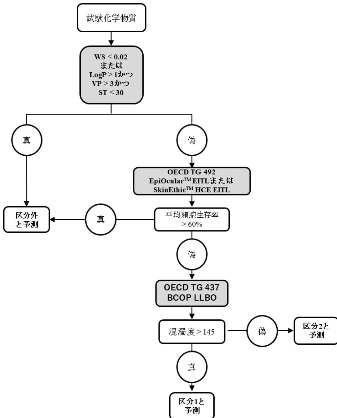
図 2.1. DAL-1 選択肢 1 の模式図。第 1 ステップ—区分外を特定する物理化学的性質の除外ルール（WS：水溶性（単位：mg/mL）か、LogP：オクタノール／水分配係数、VP：蒸気圧（単位：mm Hg）、ST：原液の表面張力（単位：dyne/cm））。第 2 ステップ—区分外の特정에用いる RhCE EITL 試験法。第 3 ステップ—区分 1 の 특정에用いる BCOP LLBO。
