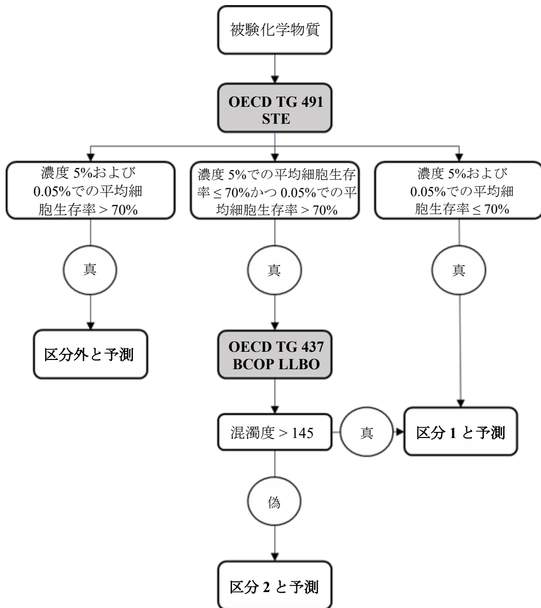
図 3.1. DAL-2 STE/LLBO 選択枝 1 の模式図 : STE 試験法から開始後、BCOP LLBO 試験法を実施
