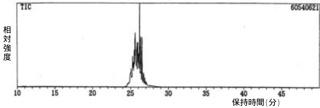
Fig.1 DINAのGC/MSクロマトグラム (1000 \mu\text{g/ml} )
