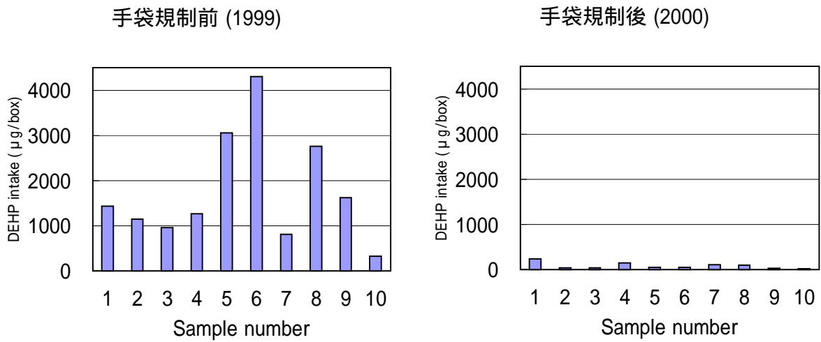
Fig.2 調理用PVC製手袋規制前後における市販弁当中のDEHP含有量(一食当たり \mu\text{g} ) 体重50kgのヒトのTDIは2000 ~ 7000 \mu\text{g/day}
