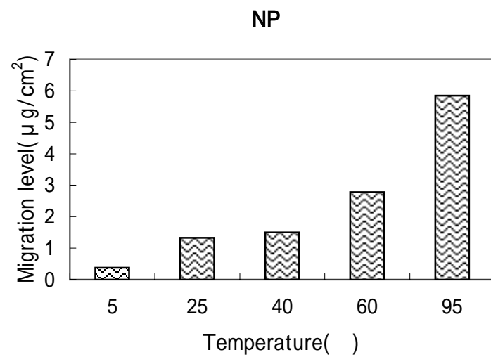
図2. 手袋3からナタネ油への溶出に及ぼす溶出温度の影響(5分間)
