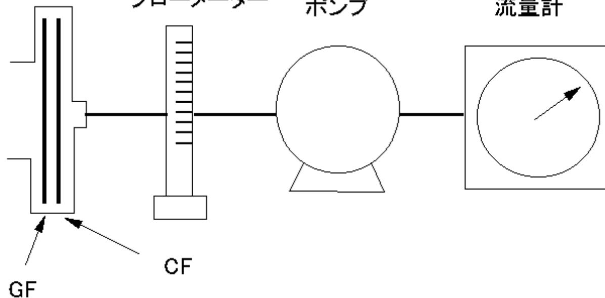
図2 可塑剤捕集装置
