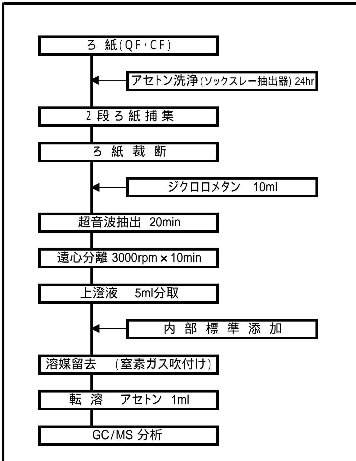
図1 可塑剤の分析フローチャート
