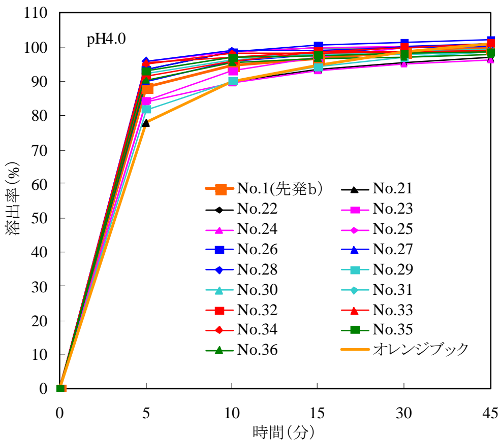
図 6 アムロジピンベシル酸塩錠 (No.21~No.36) の pH4.0 における溶出挙動
