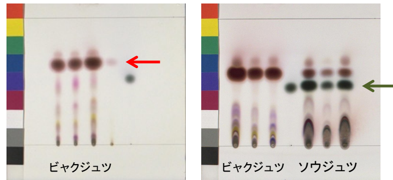
ビャクジュツの確認試験と純度試験
